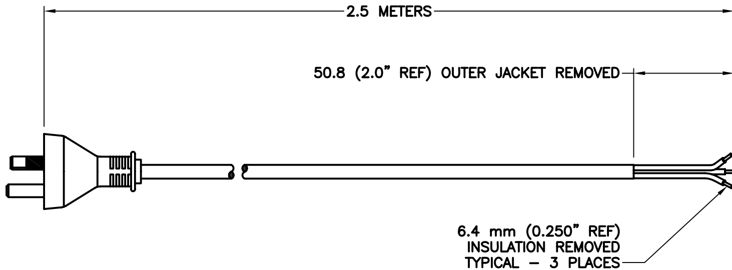
AU1-10P AS/NZS 3112
