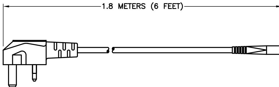
IEC 60320 C-7
