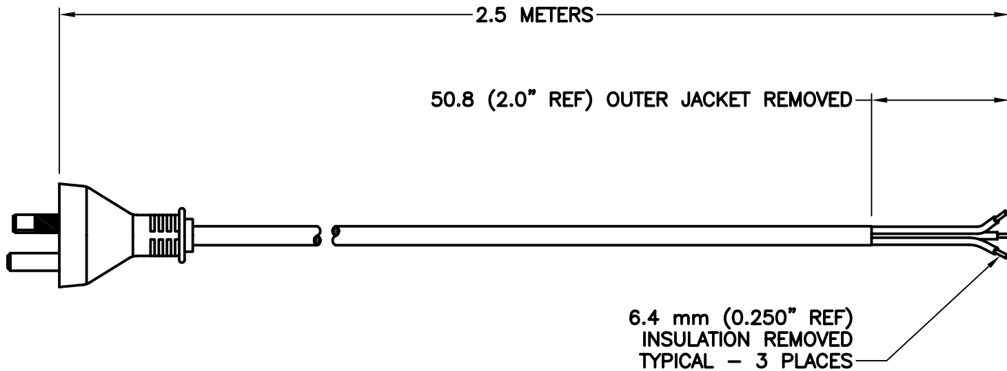
AU1-10P AS/NZS 3112
